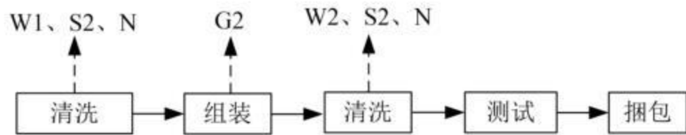
图9 流量计生产工艺流程及产污环节图
