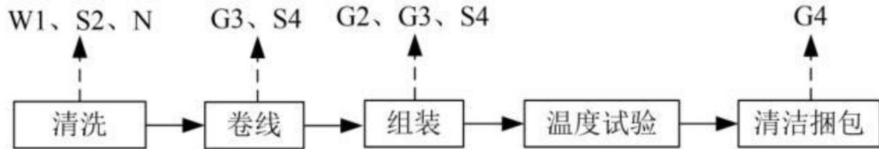
图 6 气体质量控制器传感器生产工艺流程及产污环节图
