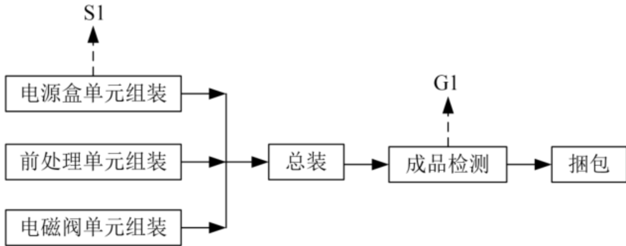
图 3 烟气分析系统生产工艺流程及产污环节图
